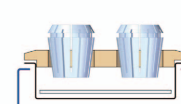
Kompletní sestava vložená do nástrojového rámu
